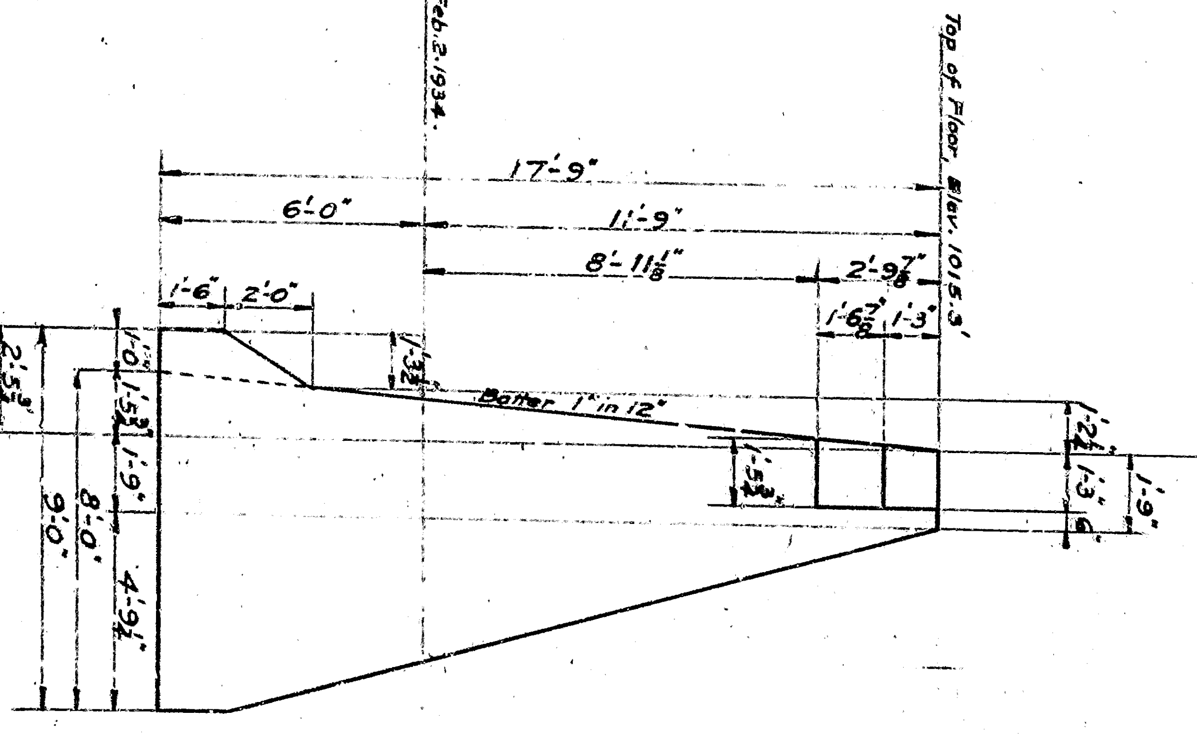
SECTION A-A
