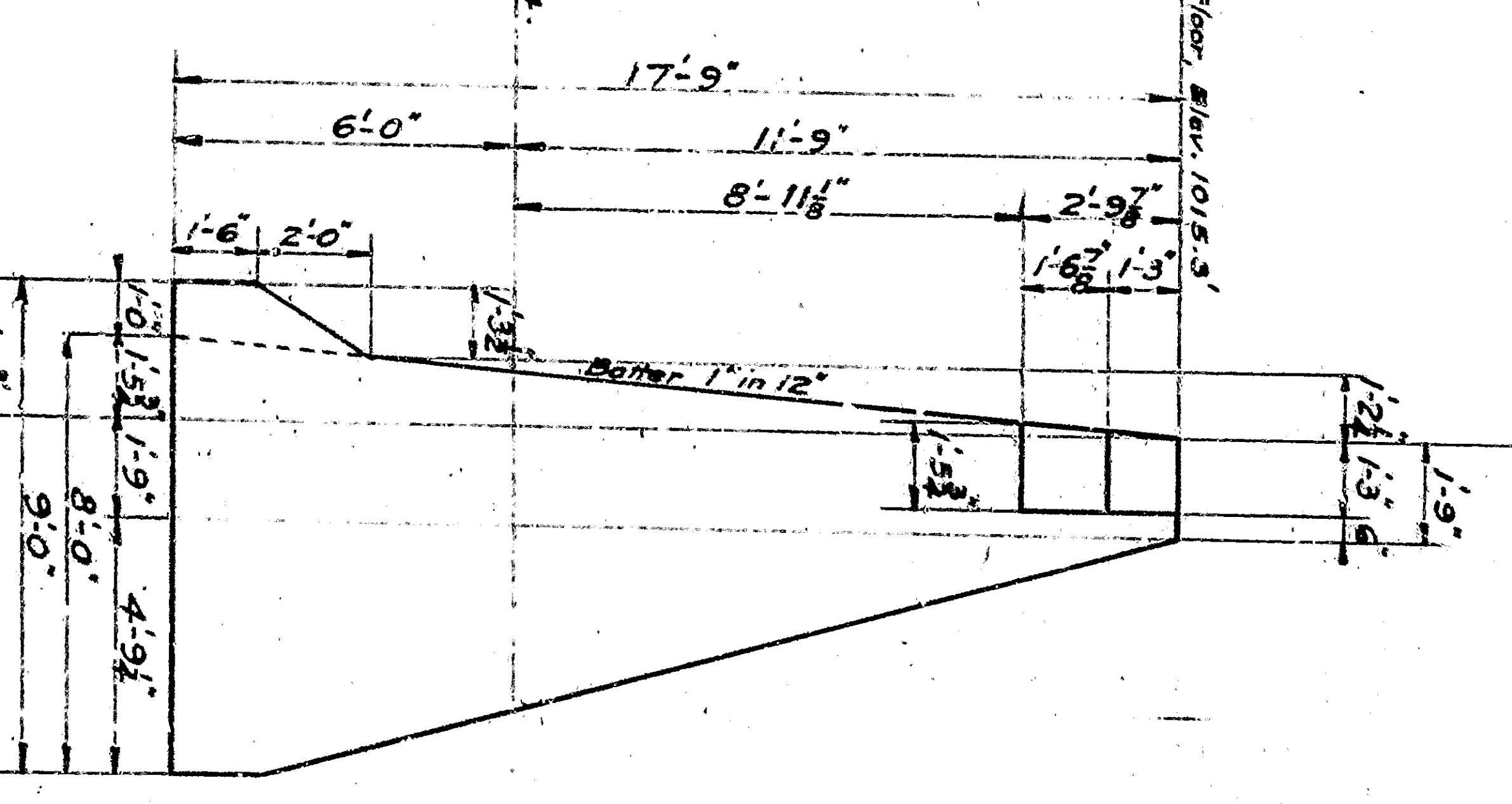
SECTION A-A
